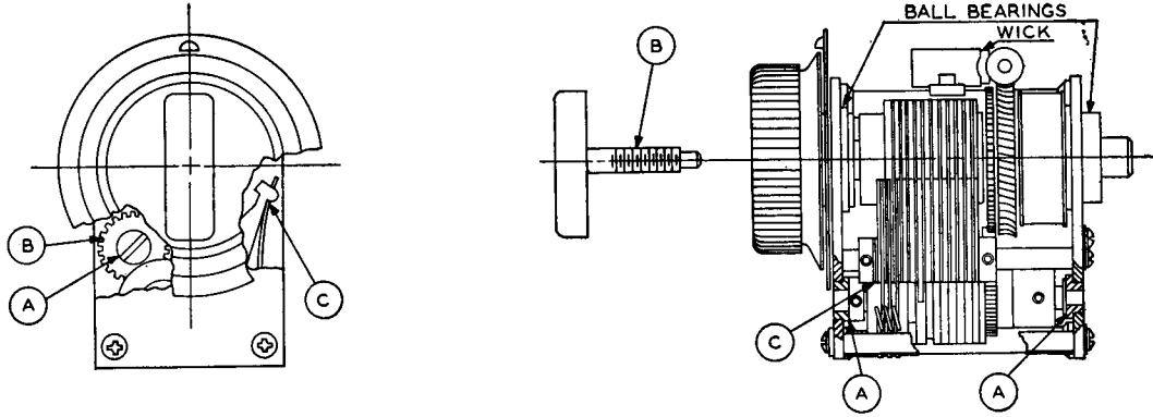
SINGLETURN UNIT
